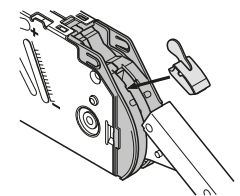
SCHEMA MONTAGGIO LIMITATORE LIMITER INSTALLATION DIAGRAM
